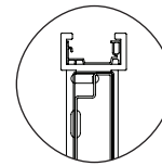
Elemento de fijación sobre panel de madera Galvanizado ML-LUM 06109T
